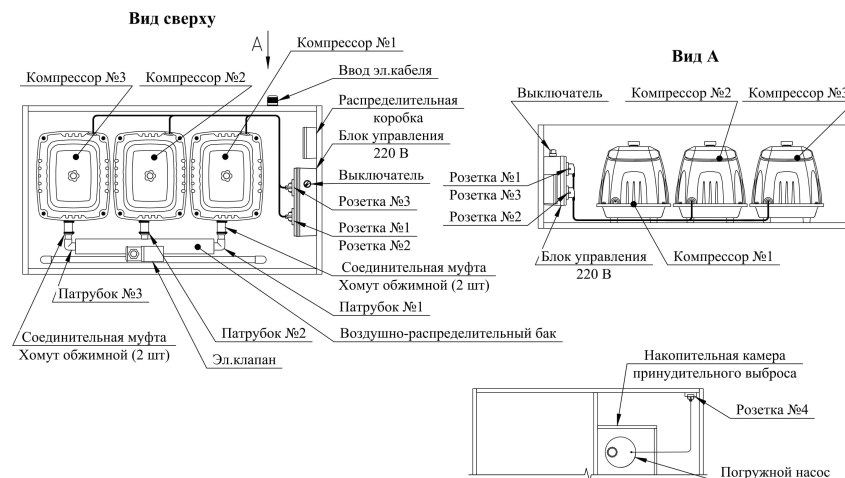
Рис. №8. УОСВ ТОПАС 75 PR с принудительным выбросом очищенной воды
