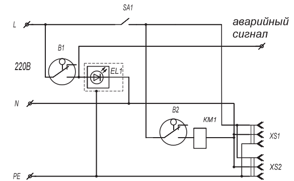
Принципиальная схема ТОПАС 40-50
