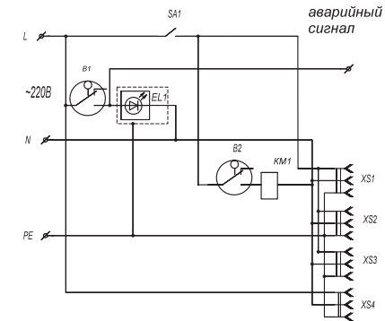
Принципиальная схема ТОПАС 150 с принудительным насосом (отсек 2)
